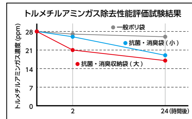
※上記4グラフ、一般財団法人カケンテストセンターによる検査結果
